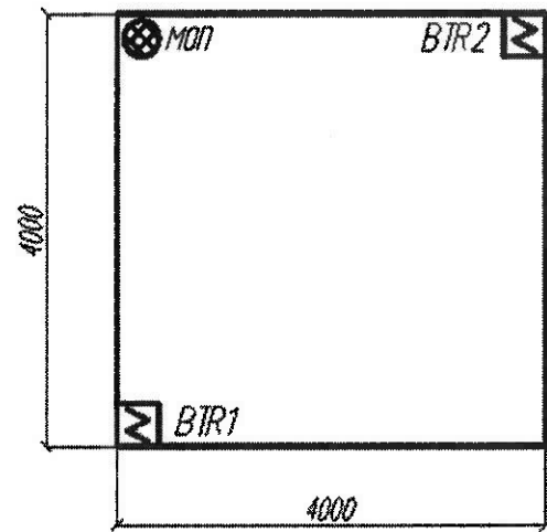
б) газовые ИП (BTR 1-2)
